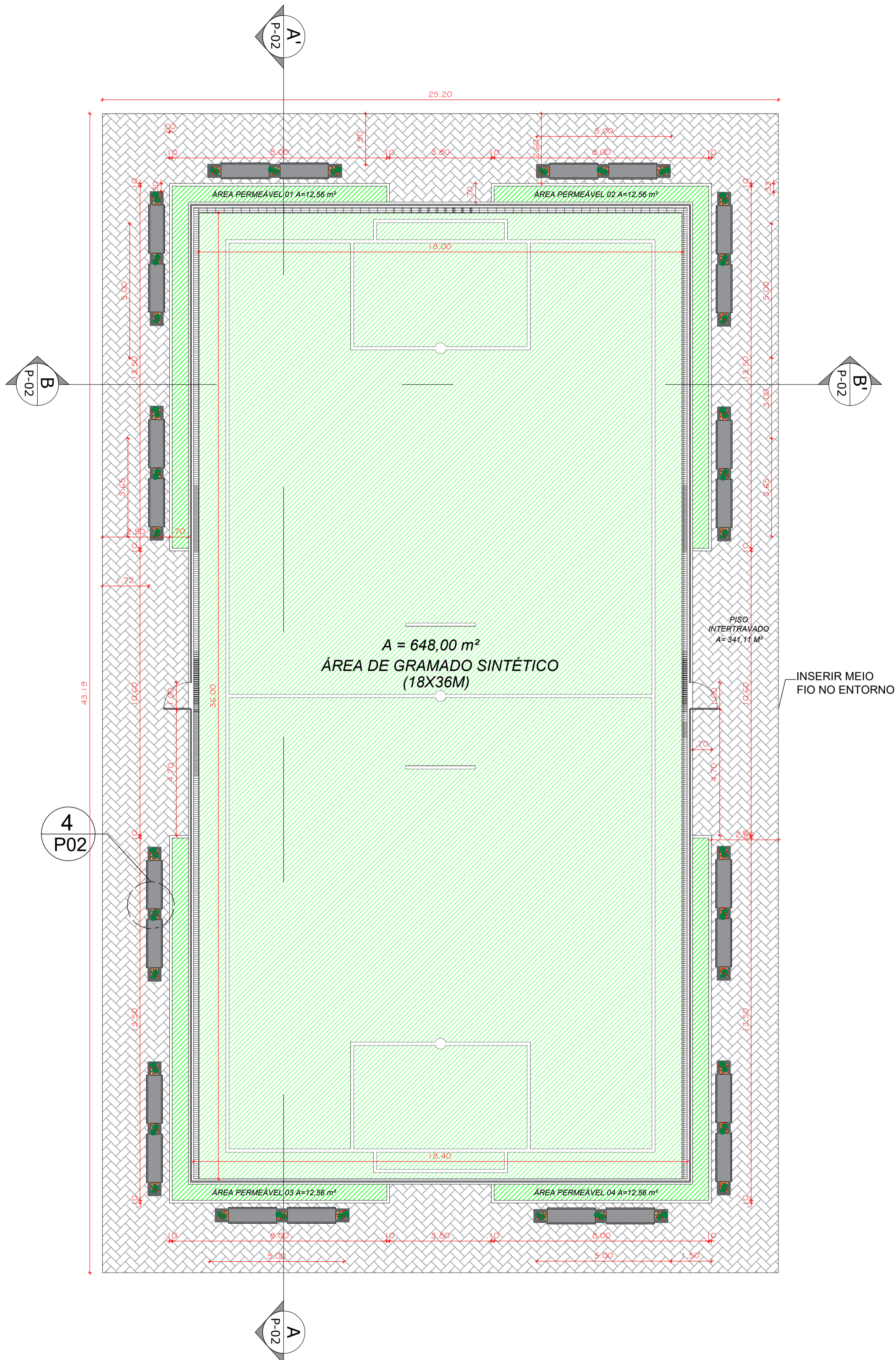
01 PLANTA BAIXA - QUADRA ESCALA: 1/100
