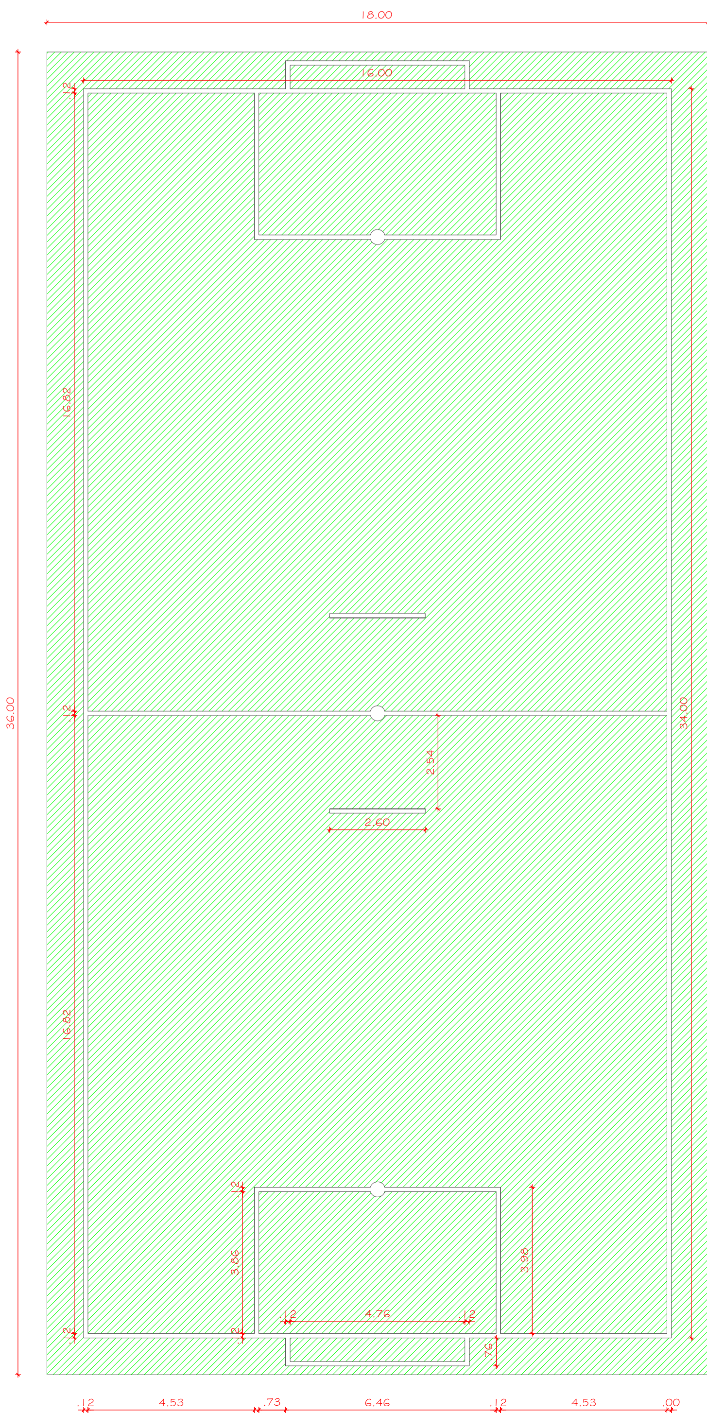
03 DETALHE MARCAÇÃO ESCALA: 1/100
