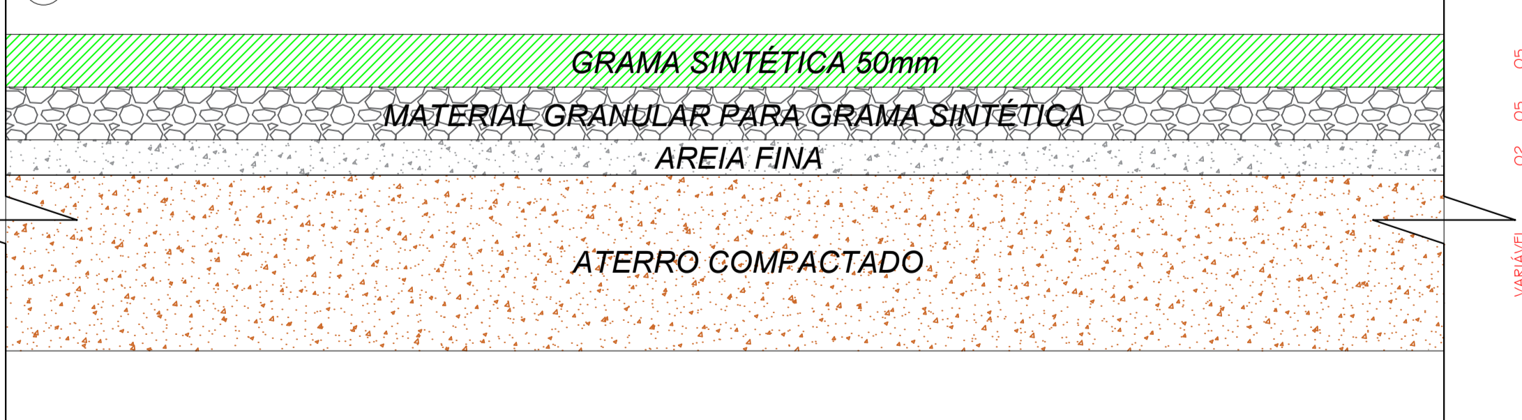
05 CORTE ESQUEMÁTICO - QUADRA SI/ESCALA
