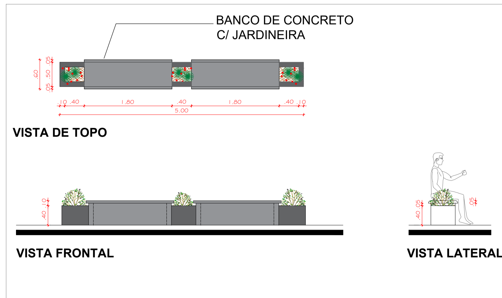
04 DETALHE MOBILIÁRIO - BANCO C/ JARDINEIRA ESCALA: 1/50
