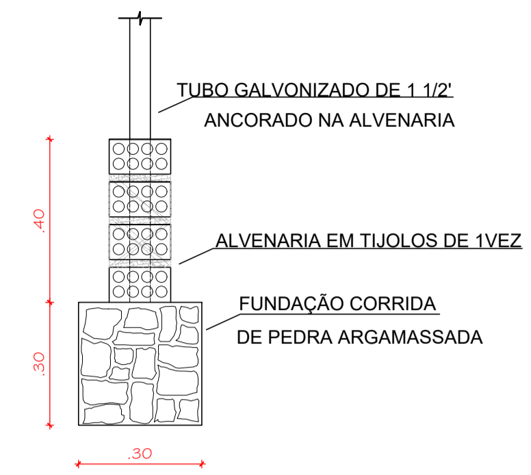
06 CORTE ESQUEMÁTICO - FUNDAÇÃO SI/ESCALA
